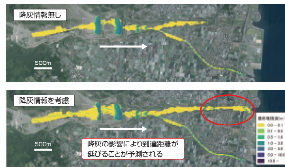
土石流シミュレーション結果
